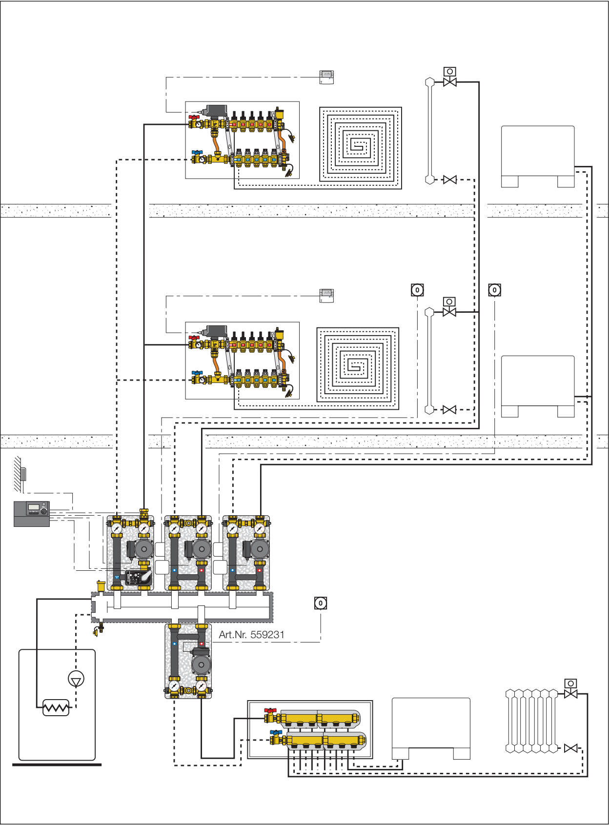
Anlage mit Standheizkessel und SEPCOLL 3+1
